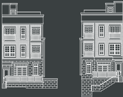
Elev. A
